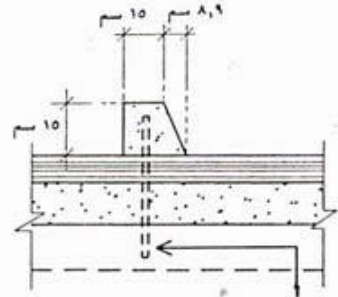
قضبان من حديد تسليح مغروسان عمودياً لتثبيت المصدرة بالأرض (البعد ١٢.٢ و ١)
